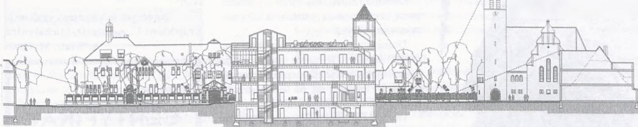
Przekrój podłużny przez teren Rynku i nowo projektowany ratusz
