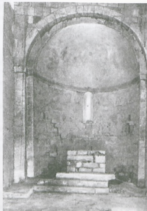
Wnętrze kościoła - długość 10,8 m, rzęso-kość 7-8 m, promień apsydy 2,3 m
