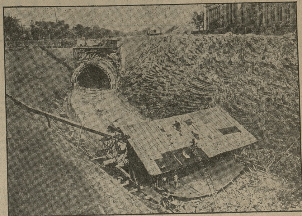
Niezwykłą regulację rzeczką Des Peres przeprowadza się obecnie w Stanach Zjednoczonych Ameryki Półn. Rzeczka ta, która corocznie wylewała na wiosnę i jesienią, wyrządzając znaczne szkody, zniknie pod ziemią w olbrzymim tunelu.
