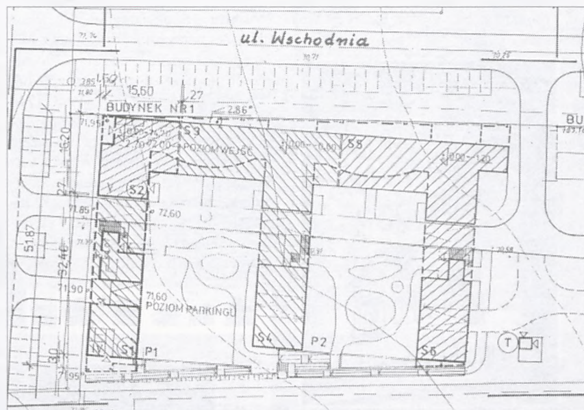
Ryc. 2. Położenie i układ budynku przy ulicy Wschodniej
