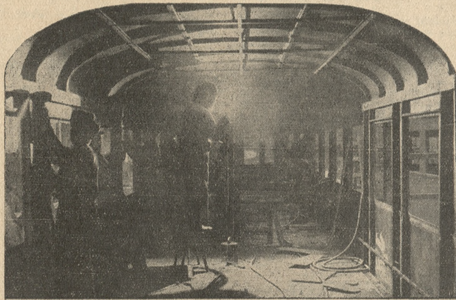
WNĘTRZE POLSKIEJ TORPEDY PODCZAS MONTAŻU
