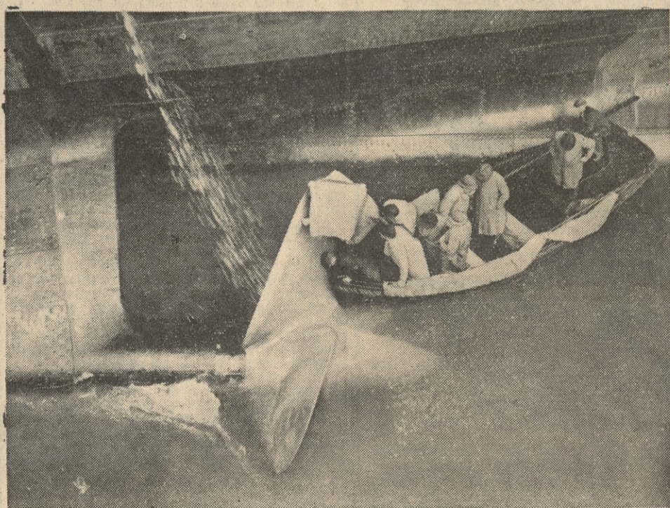
Inżynierowie stoczni w Southampton dokonali przeglądu śrub transatlantyka angielskiego „Queen Mary”, który wrócił z Ameryki. Cztery nowe śruby będą odtąd poruszały olbrzyma.
