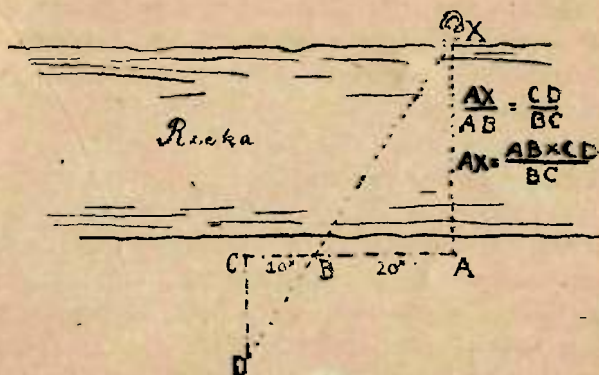
Pomiar szerokości
