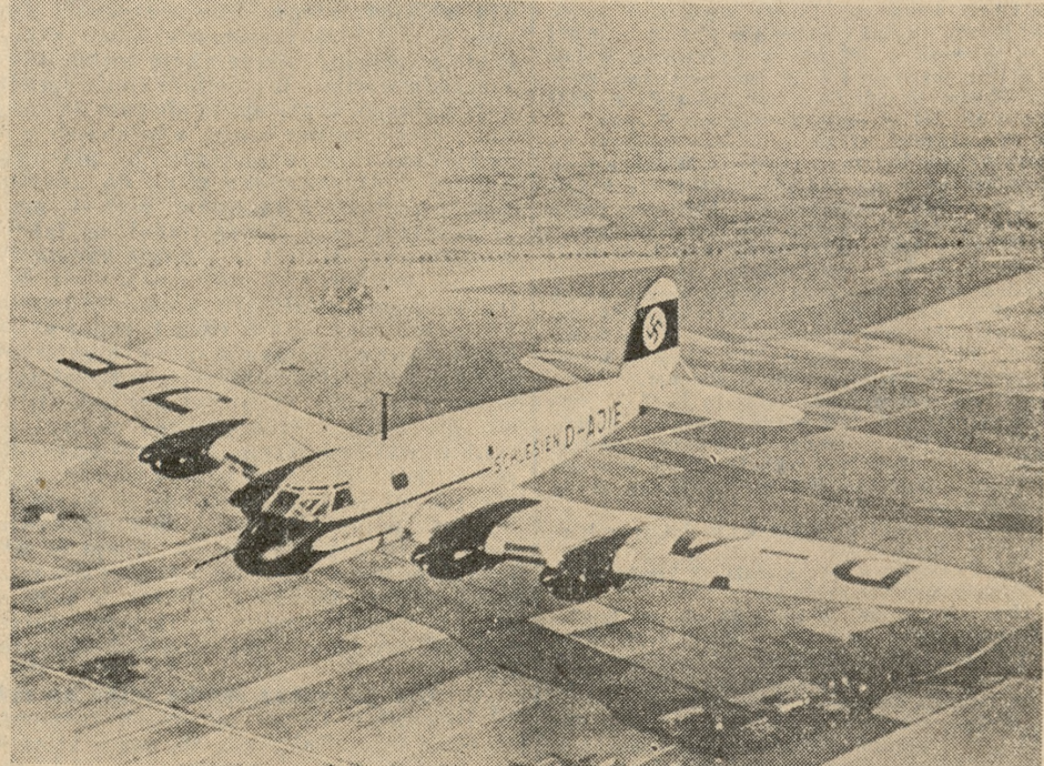
Do lotów transatlantycznych wybudowali Niemcy nowy czteromotorowiec pocztowy Heinkel — He 116. Ołbrzym ten może przy 4 ludziach obsługi i 550 kg poczty przebyć przy szybkości 300 km. na godz. bez lądowania przestrzeń 4.500 km. Długość samolotu wynosi 13,7 m, a rozpiętość skrzydeł 32 m.
