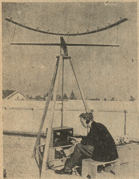
Amerykańska ultrakrótkofalowa stacja odbiorcza dla fal 1,5 m służy do łączności z balonem meteorologicznym. Nadajnik przekazujący automatycznie wskazania przyrządów meteorologicznych, waży tylko 420 gramów.
