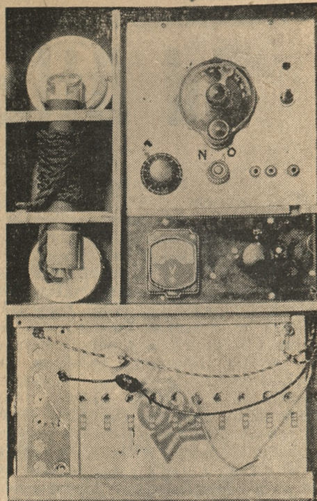
Przenośna stacja nadawczo-odbiorcza U. K. F. — P. K. K. Po prawej u góry aparatura nadawczo-odbiorcza, poniżej instrumenty pomiarowe, po lewej słuchawka-mikrofon, na dole bateria anodowa.
