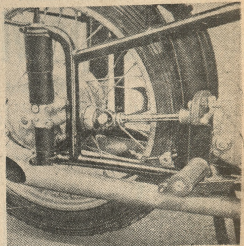
Resorowanie koła tylnego motocykla wyścigowego BMW posiada sprężyny umieszczone w rurze rozsuwającej się na kształt teleskopu.
