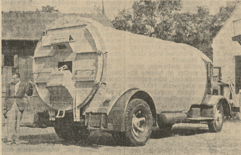
Nowoczesny olbrzymi samochód-śmieciarka, pojemności 10—15 ton, przeznaczony do mechanicznego, bezpylnego wywożenia śmieci.
