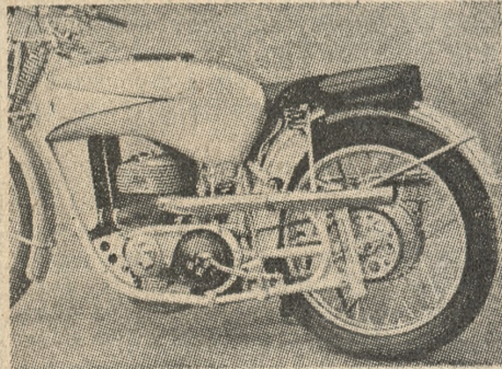
Resorowanie tylnego koła w motocyklu wyścigowym DKW. Sprężyny umieszczono w rurze służącej jako prowadzenie.
