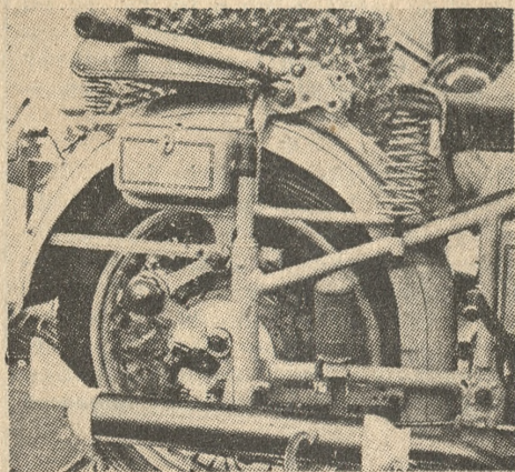
Włoski motocykl wojskowy z resorowanym kołem tylnym. Sprężyny w rurze prowadzącej przestawiają się samoczynnie na większe obciążenie z chwilą podniesienia uchwytów tylnego siodełka.
