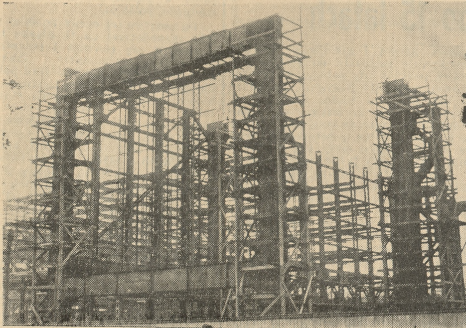
Fragment potężnych konstrukcji żelaznych przyszłego dworca centralnego w Warszawie, który już w przyszłym roku oddany będzie częściowo do użytku publicznego.
