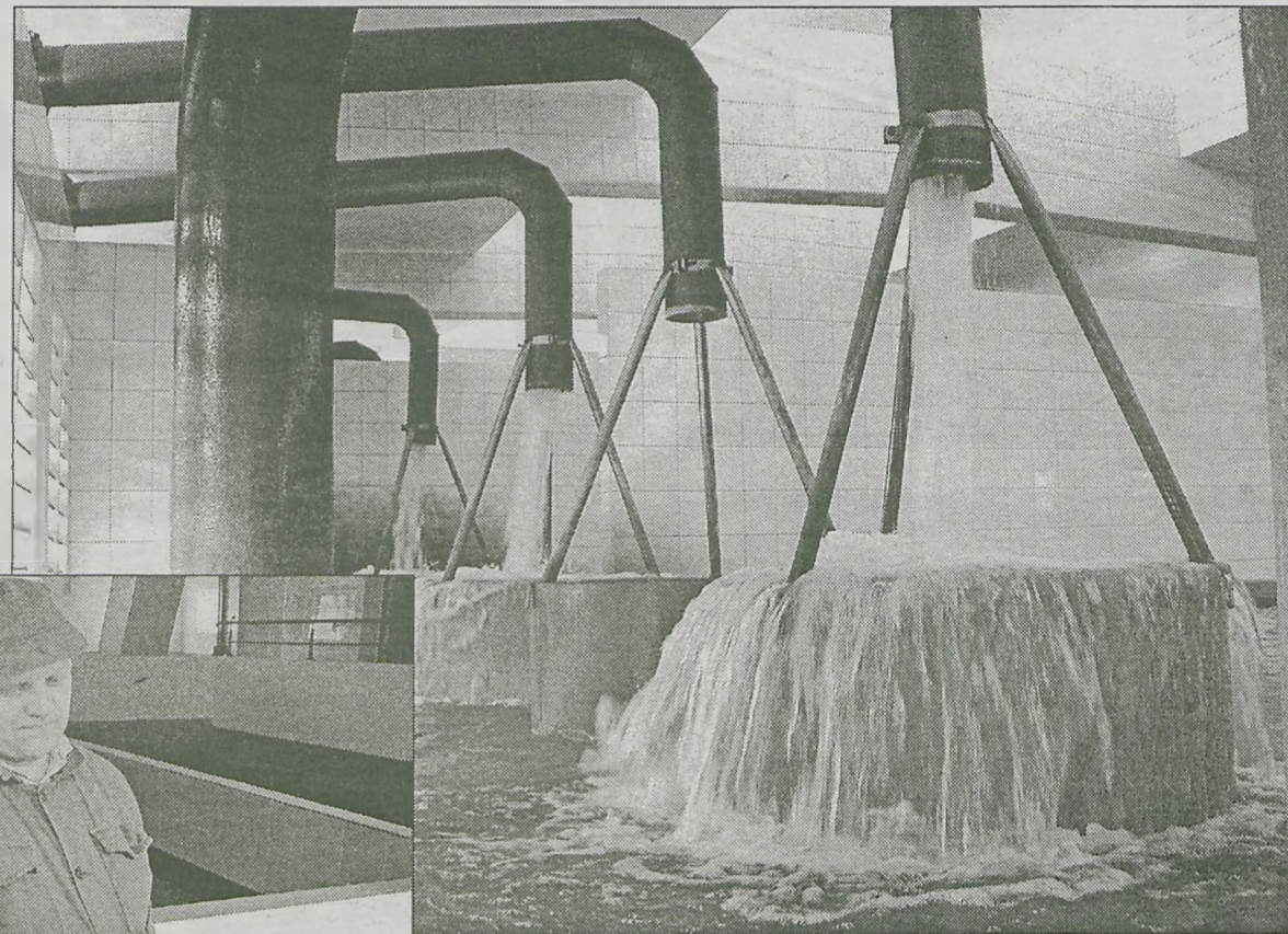
Woda ze studni głębinowych trafia do napowietrzalni
