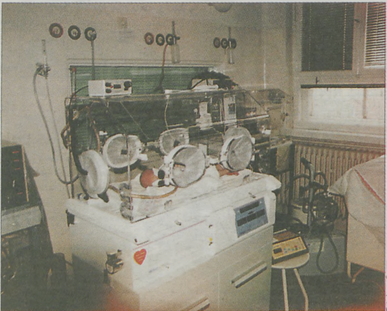
Inkubator służyć będzie noworodkom przedwcześnie urodzonym, zapewniając im odpowiednią temperaturę, wilgotność i izolację od środowiska zewnętrznego
