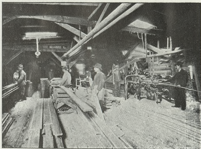
Wnętrze fabryki w Poznaniu.
