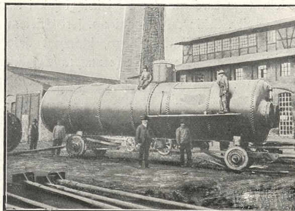
Kocioł dla wodociągów w Poznaniu, zbudowany 1903 r.
