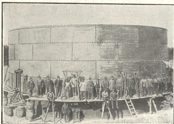
Cysterna do nafty w Starołęce, 2,700.000 ltr.
