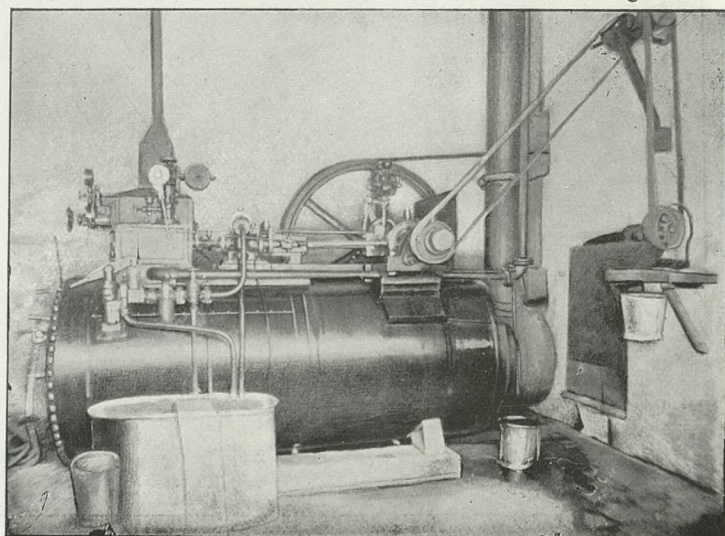
Motor parowy.
