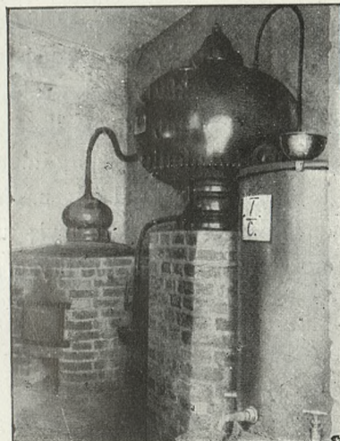
Francuskiego wyrobu aparat do wypalania koniaku.
