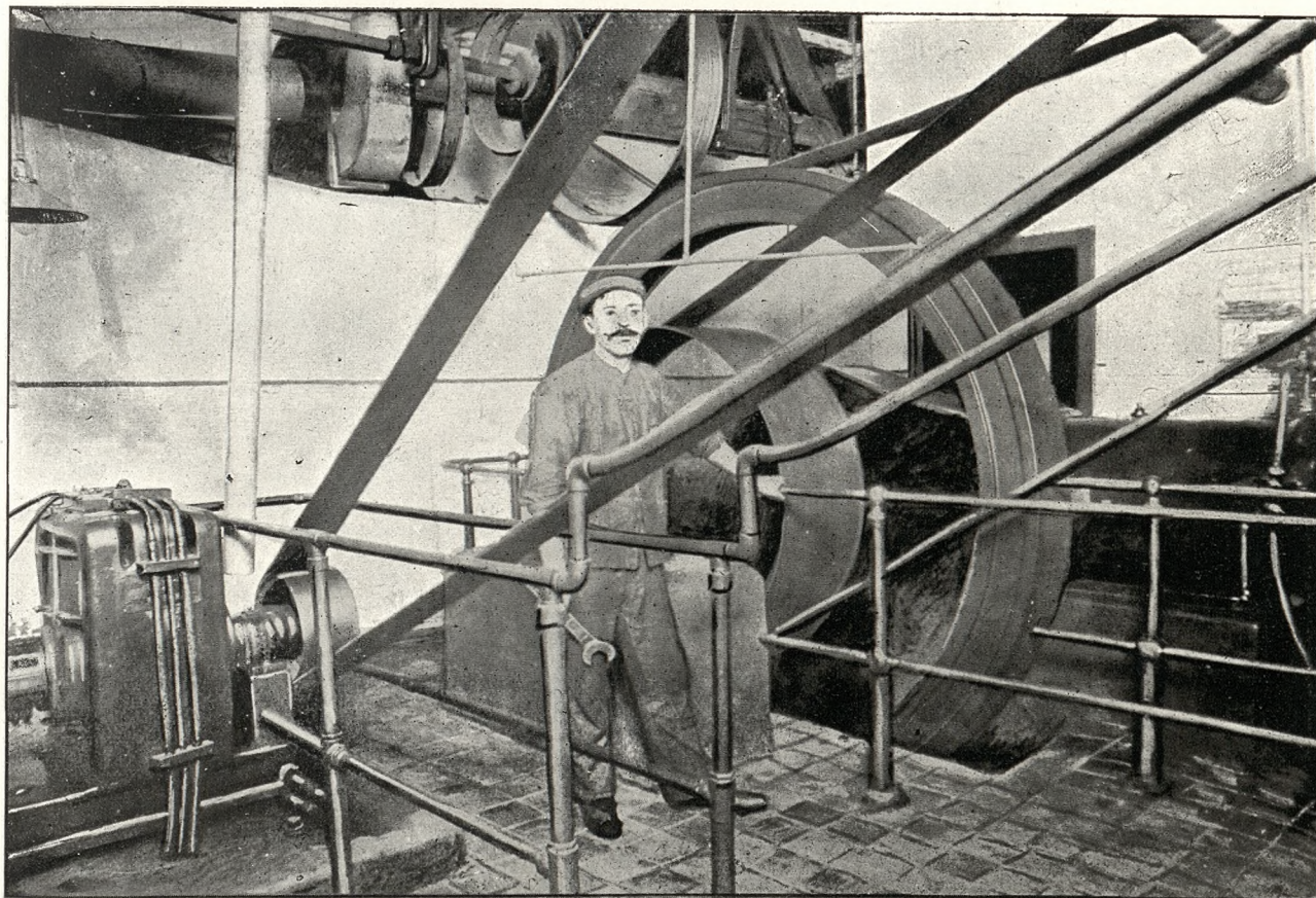
Dynamo i motor gazowy.
