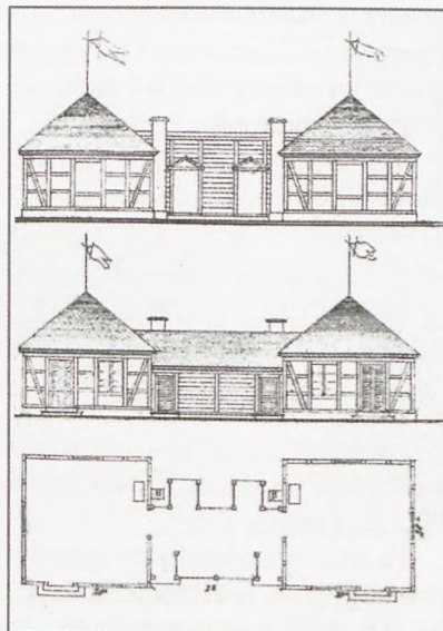
11. Plan budynku strzałowni na starej strzelnicy (APP).
