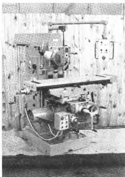
Frezarka FWF 32 z przyrządem do dłutowania kanałków oraz wielowypustów
