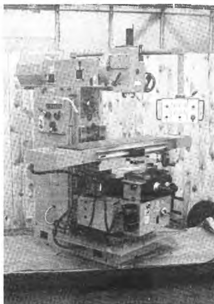
Frezarka FWR 40J2 wspornikowa pozioma uniwersalna
