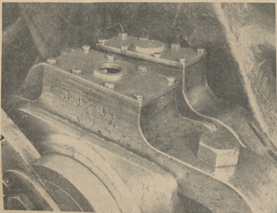
Oliwiarka parowozowa, wynalazek Fr. Śliwińskiego, maszynisty kolejowego z Poznania, dająca zaoszczędzenie smaru.
