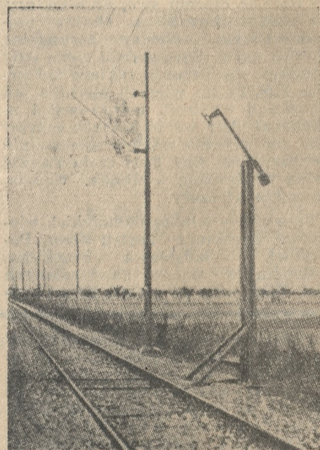
Odcinek toru ubezpieczony automatycznym urządzeniem Koflera podczas prób dokonanych przez Towarzystwo Milano-Nord pod Florencją.
