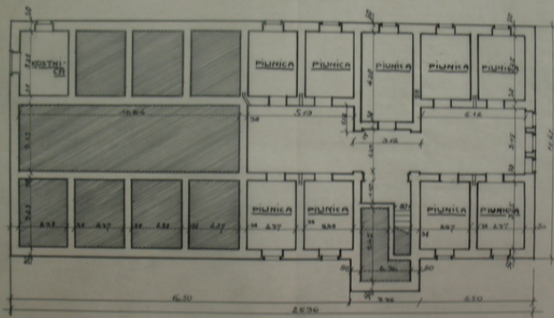
RZUT PIWNIC
