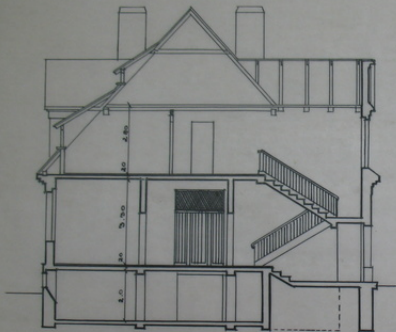
PRZEKRÓJ POPRZECZNY
