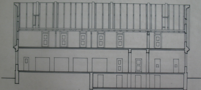
PRZEKROJ PODŁUŻNY.
