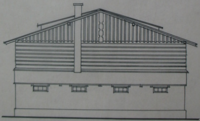
WIDOK BOCZNY.
