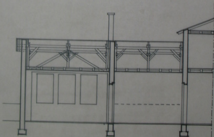
PRZEKROJ G-H.
