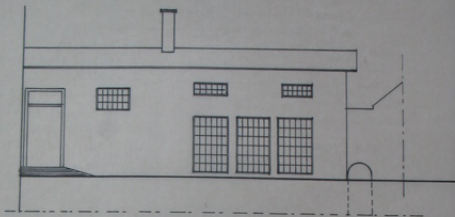
WIDOK TYLNY
