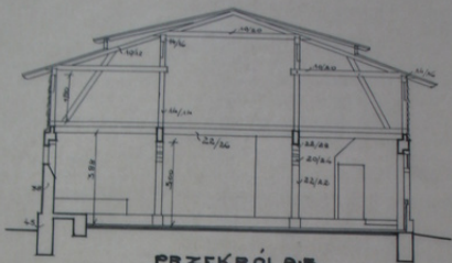
PRZEKROJ A-B.
