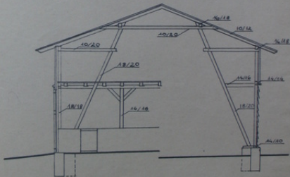
PRZEKROJ POPRZECZNY
