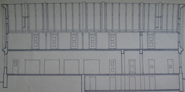
PRZEKROJ PODŁUŻNY.
