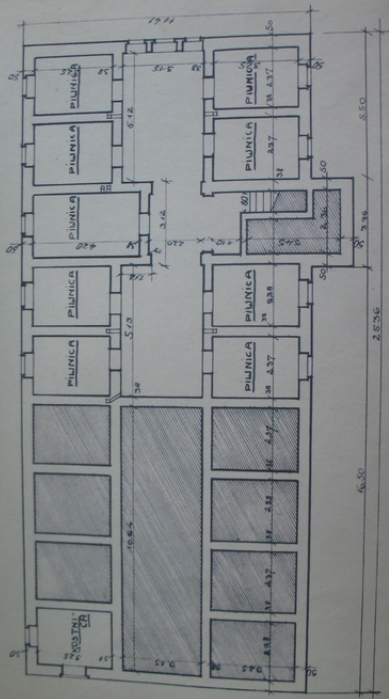
RZUT PIWNIC.
