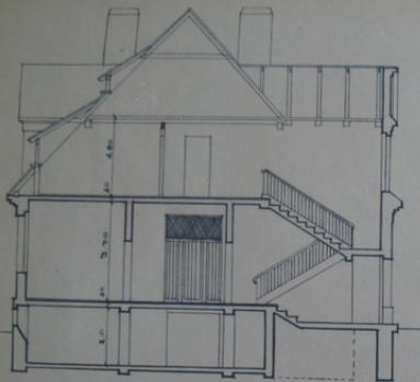
PRZEKROJ POPRZECZNY
