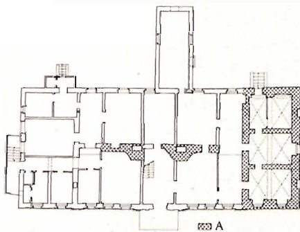
Rzut pałacu: A – najwcześniejsza faza budynku
