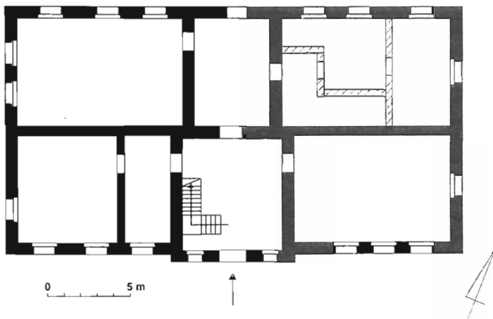
Rzut dworu barokowego w Starym Tomyślu
