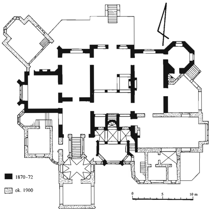
Rzut zamku w Wąsowie
