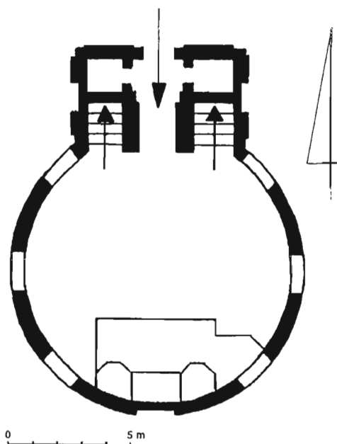
Rzut kaplicy w Wąsowie
