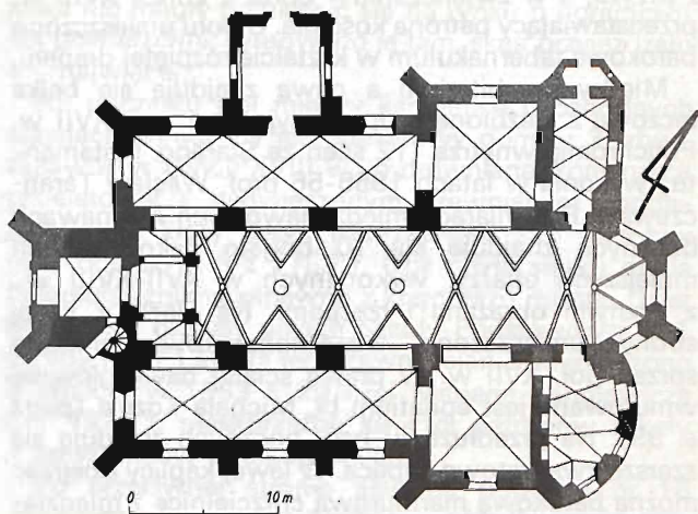
Rzut kościoła farnego
