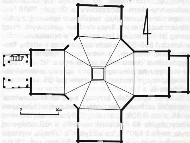
Rzut kościoła św. Fabiana i Sebastiana
