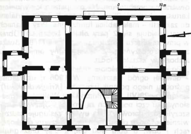
Pałac – rzut I piętra
