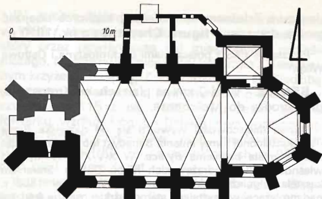
Benice - rzut kościoła św. Mikołaja
