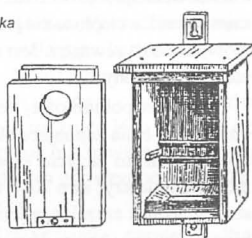
Ryc. 4. Skrzynka zwykła w przekroju.
