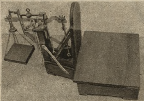
R. 1. Waga dziesiętna nie wykleszczona.
