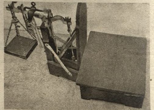
R. 2. Waga dziesiętna wykleszczona. Wykleszczenie znajduje się w pobliżu języków wagi.
