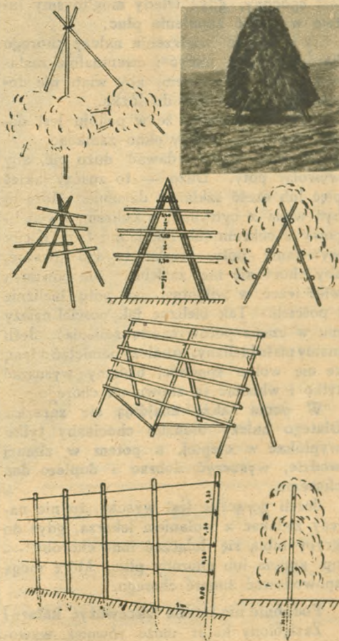
Przyrządy do suszenia lucerny
