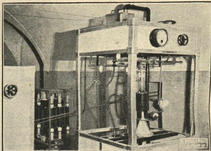
Oscylator główny
