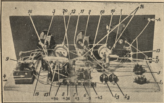
Fig. 13. Wnętrze stabilidyny. A — zacisk anteny. Z — ziemi, 1 — kondens. na 500 cm. C. 2 i 3 kondens. po 200 cm. C. 4 — sprzęgacz na 2 cewki, 5, 9, 20 — trzy z pośród podstawek do lamp, 10, 11, 12 reostaty 13 — przełącznik, 14 i 15 — kondensatory stałe, 16 i 19 — transformatory, 17 i 18 — kondensatory neutralizujące, L_1 , L_2 i L_3 podstawki do cewek odpowiednio do schematu na fig. 12.
