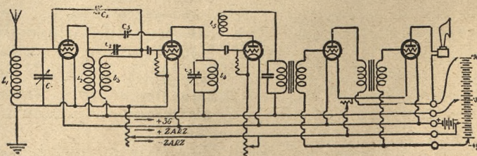
Fig. 12. Schemat Stabilidyny.
