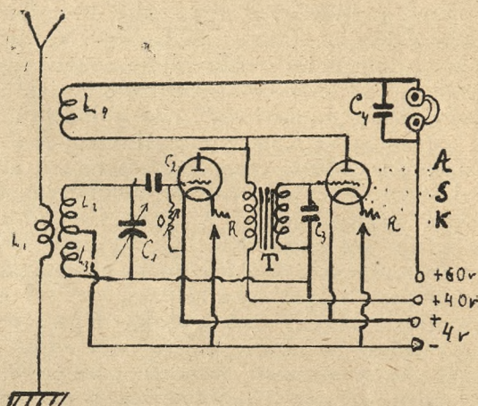
Fig. 11. Schemat A - anoda, S - siatka, K - katoda.
