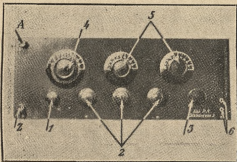
Fig. 14. Płyta rozdzielcza stabilidyny. A — zacisk antenowy, Z — uziemienia, 1 — przełącznik na 4 i 5 lamp, 2 — reostaty, 3 — gałka sprzęgacza, 4 — kondensator zm. 500 cm. C. 5 kondensatory zm. po 200 cm. C. 6 — tulejki telefonu.
