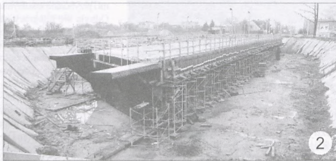
Wiadukt WD2 - ul. Kościuszki
