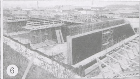
Po wschodniej stronie torów Lubon-Staroleka budowa „przesuwnej obudowy tuneli”
